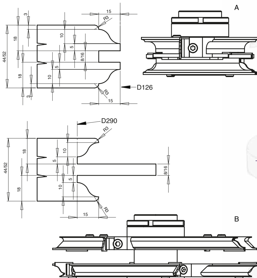
GRUPPO DI PORTACOLTELLI PER PORTE E PORTONCINI 44/52 MM GROUP OF CUTTERS FOR DOORS AND MAIN DOORS 44/52 MM
